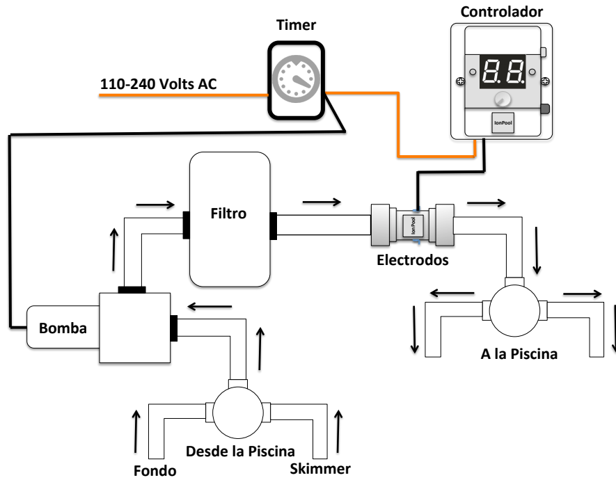
Figura 2 Esquema de conexión
