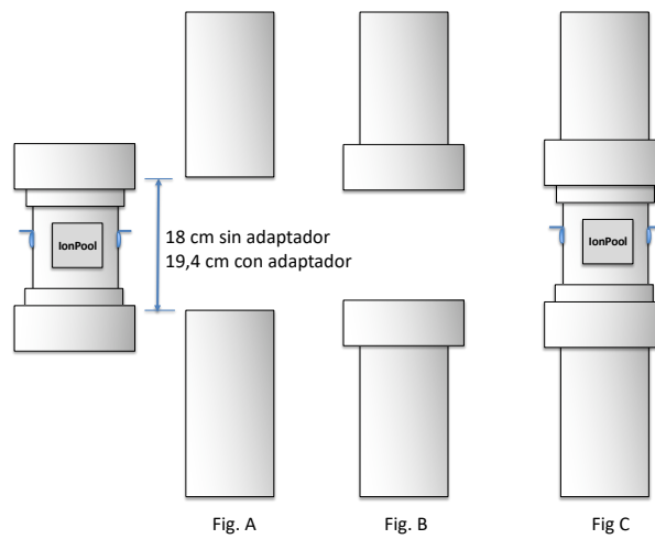
Figura 3 Instalación del electrodo
